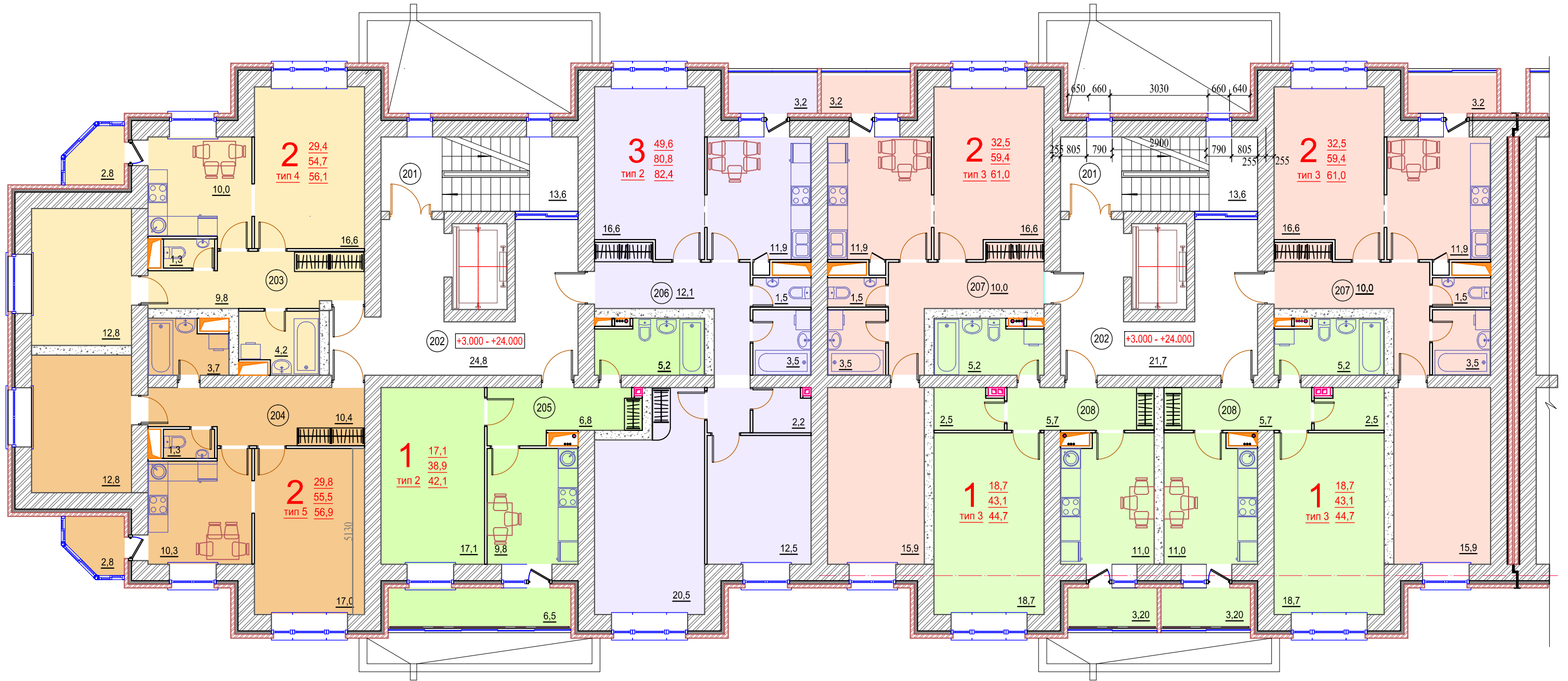
Блок А. План типового ( 2- 9 ) этажа
