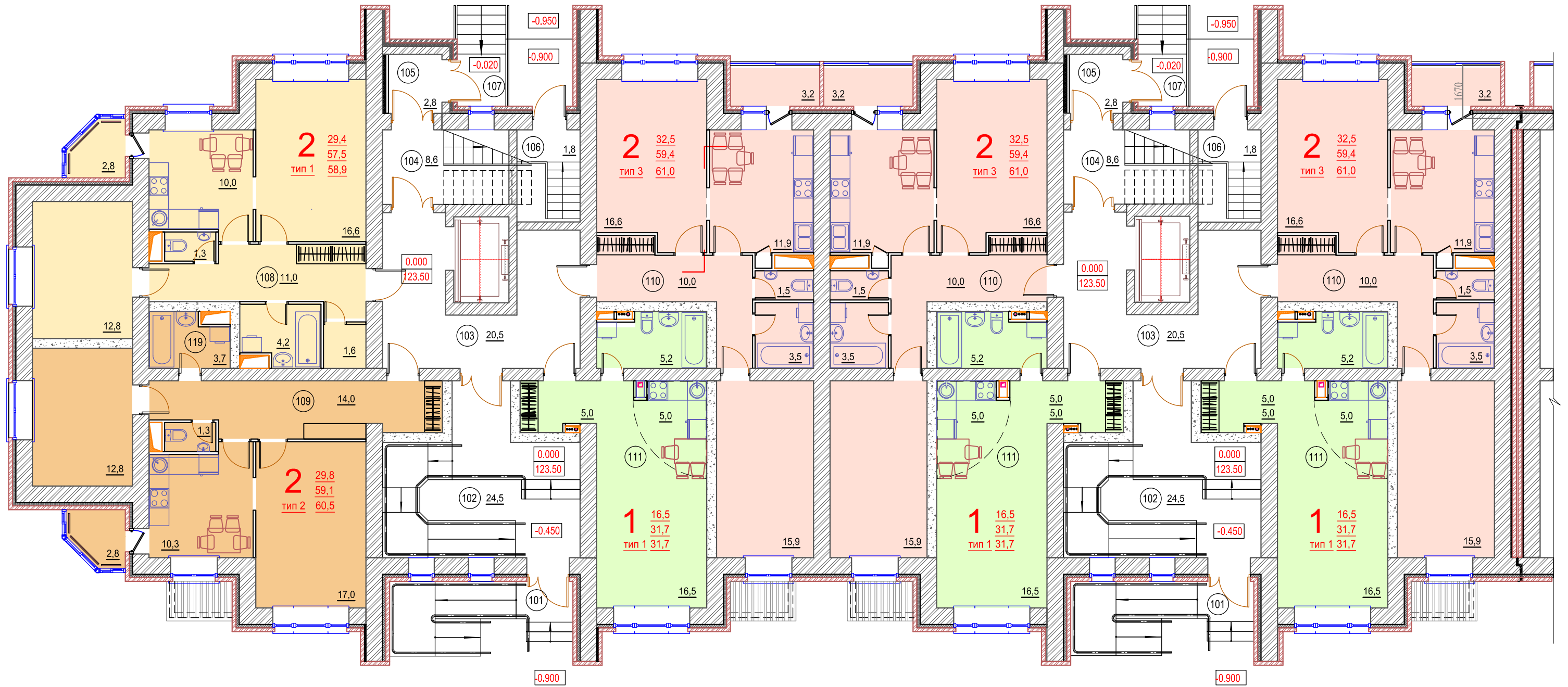
Блок А. План 1 этажа
